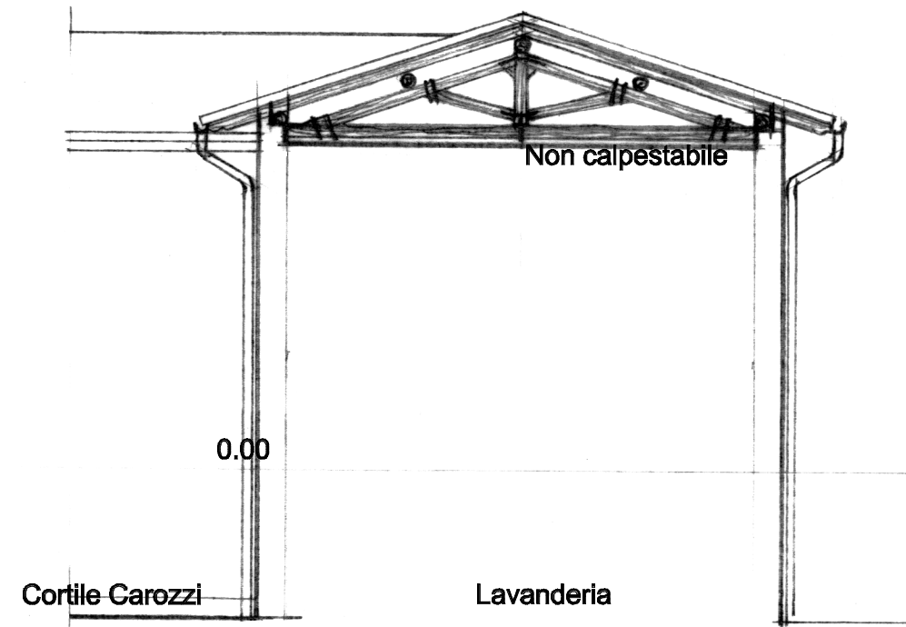
SEZIONE B-B
