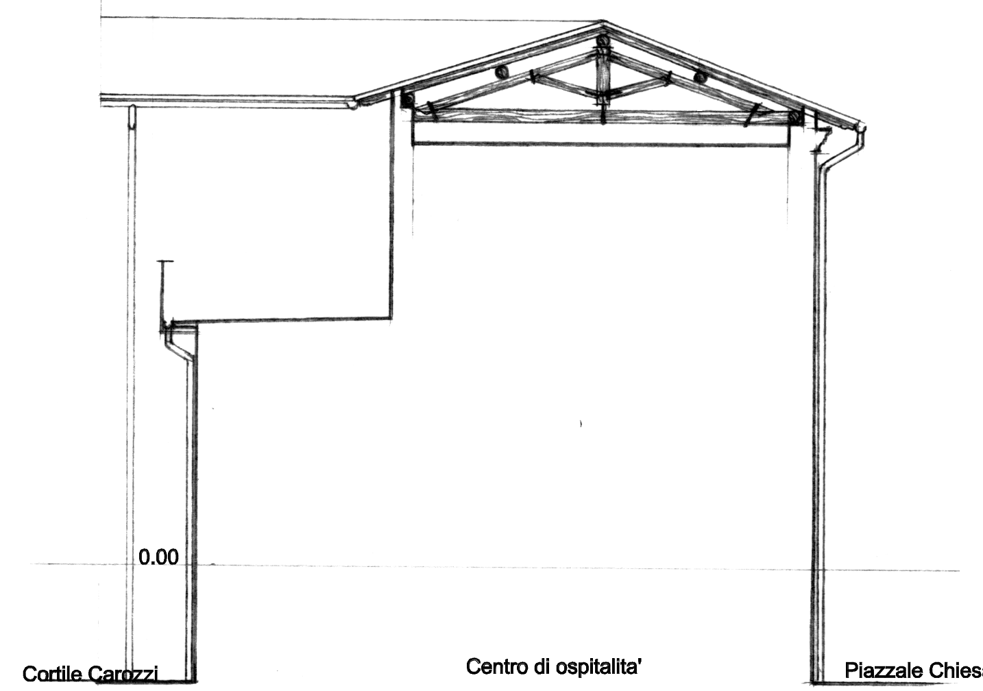
SEZIONE D-D
