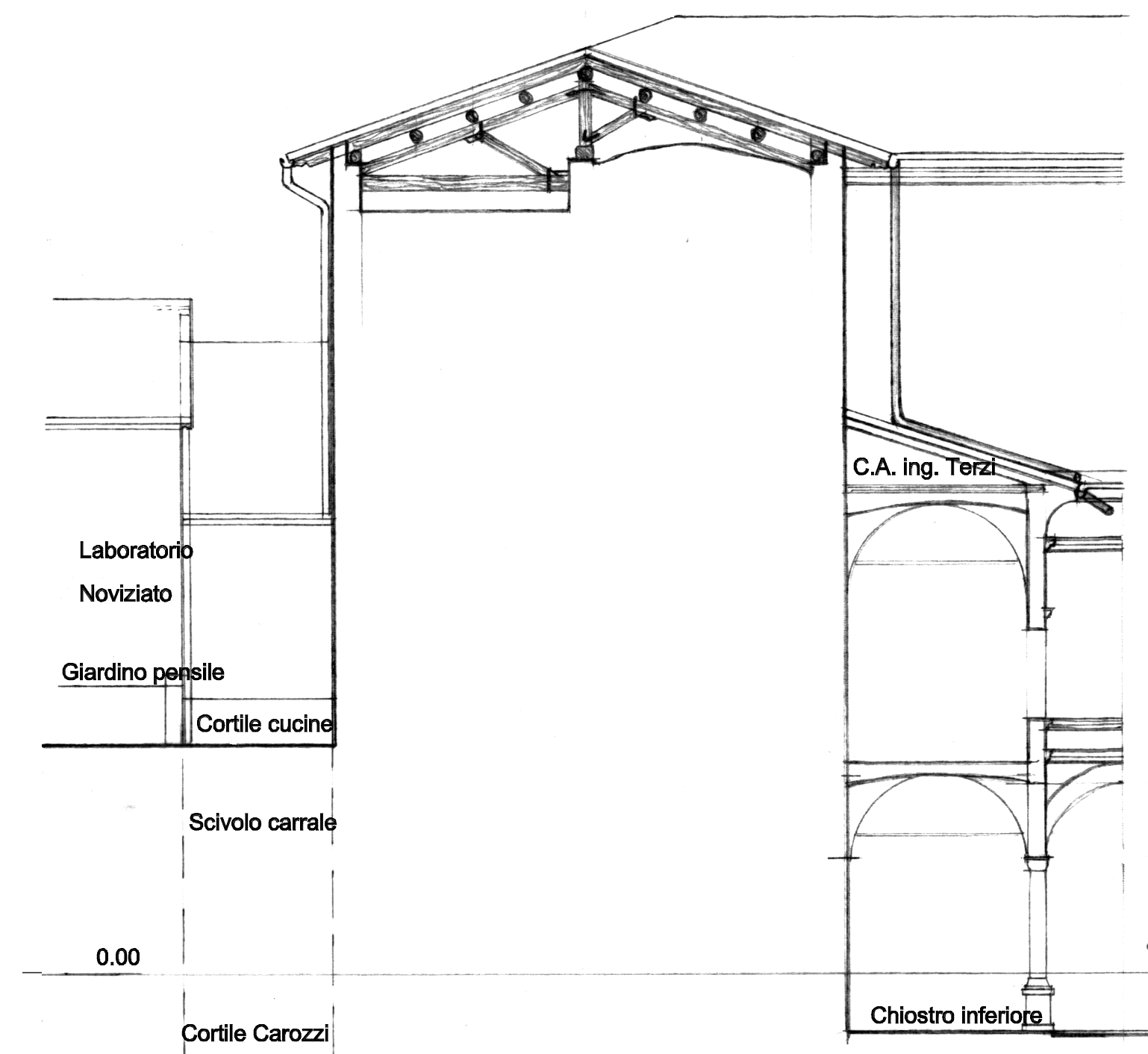
SEZIONE G-G
