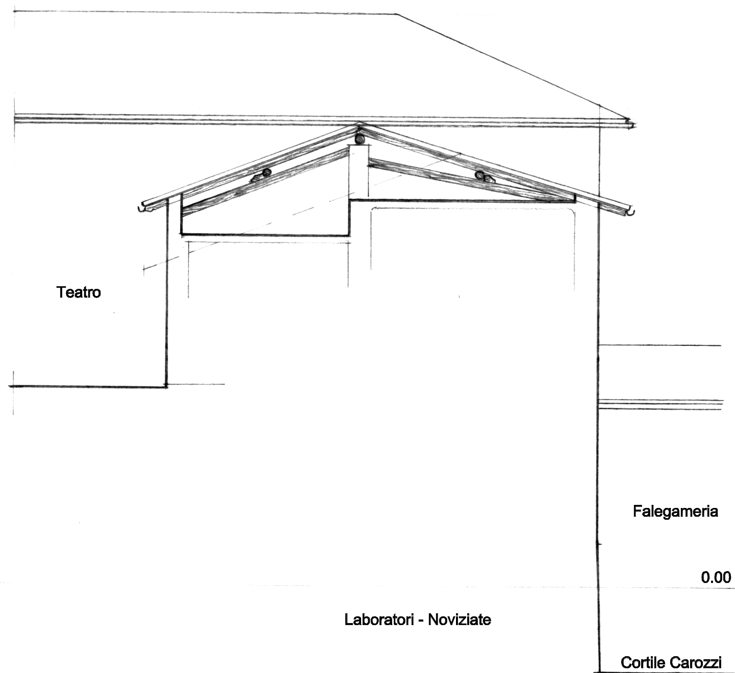
SEZIONE E-E
