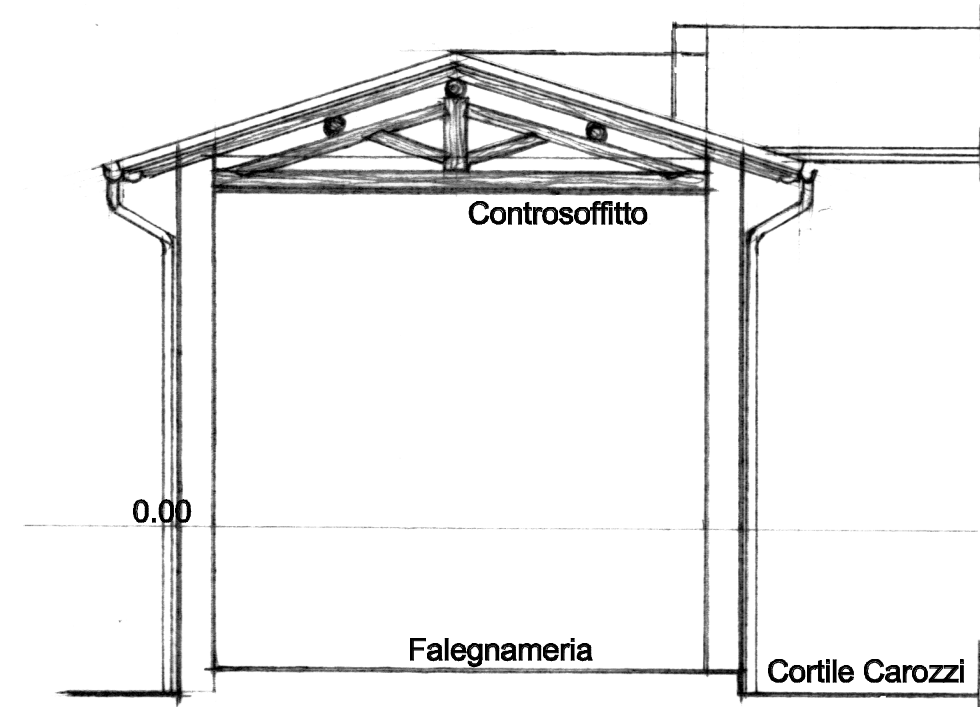
SEZIONE A-A
